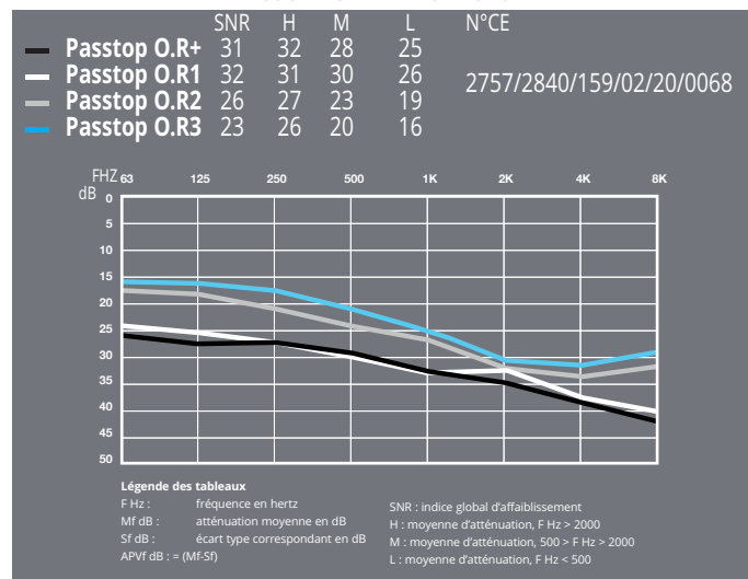
COURBES D'ATTENUATIONS
