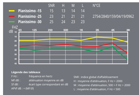
COURBES D'ATTENUATIONS
